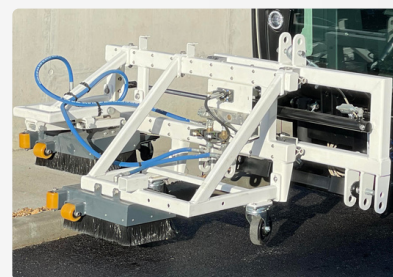
Rampe Dyn'
